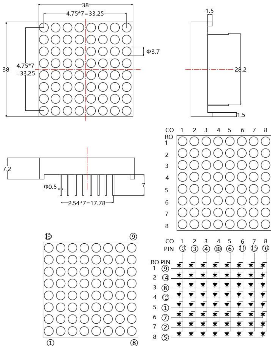
数码管显示及引脚位置图
