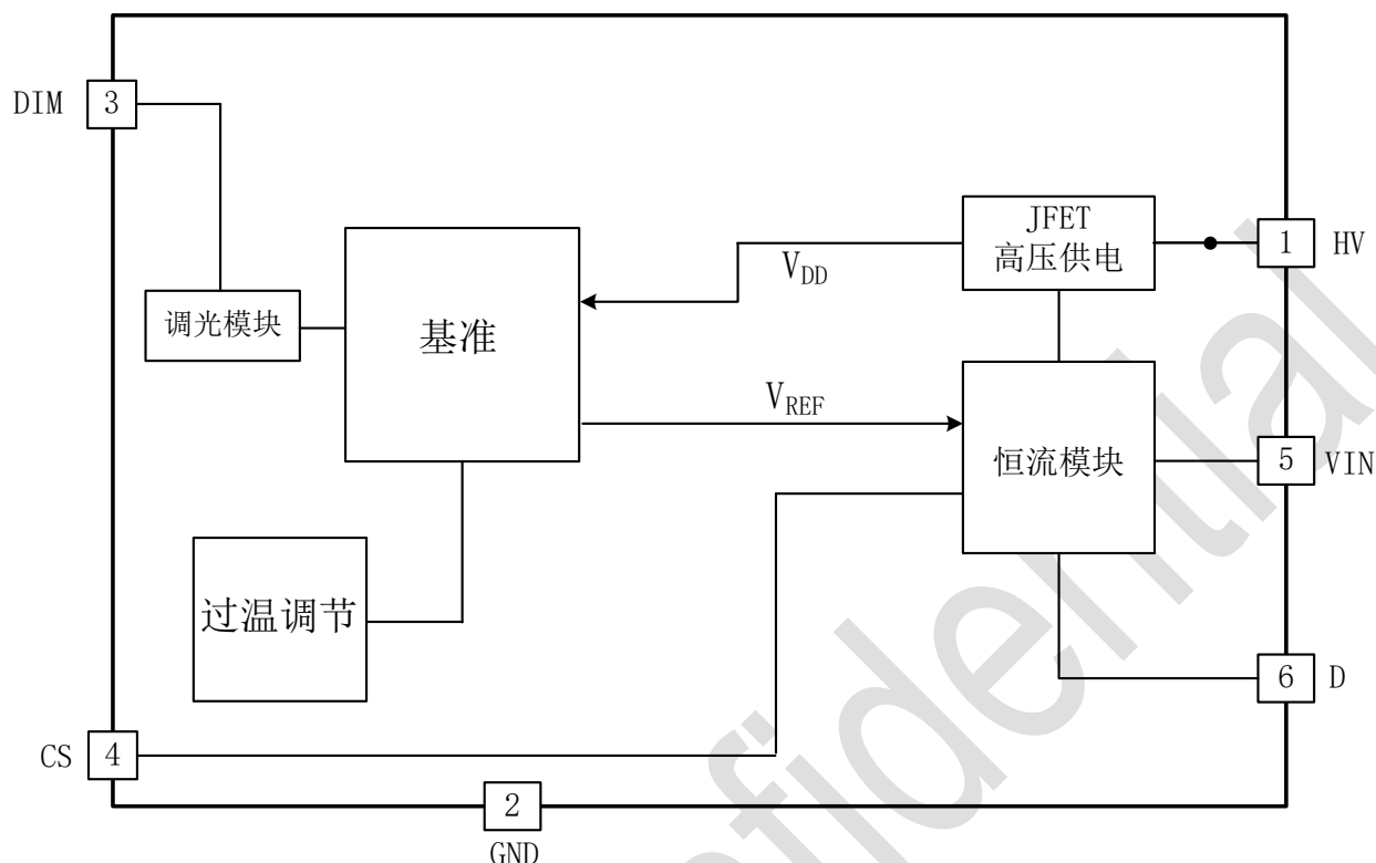
图 3 BP5176GC 内部框图
