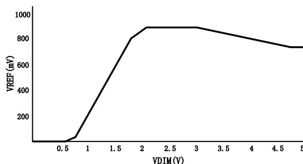
图 4 VDIM 调光曲线
