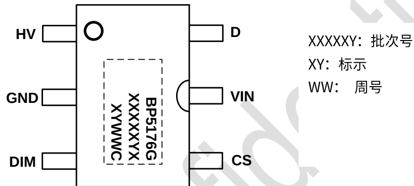
图 2 管脚封装图
