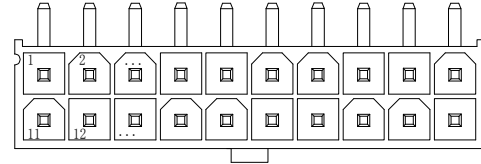
2x10 Pin
