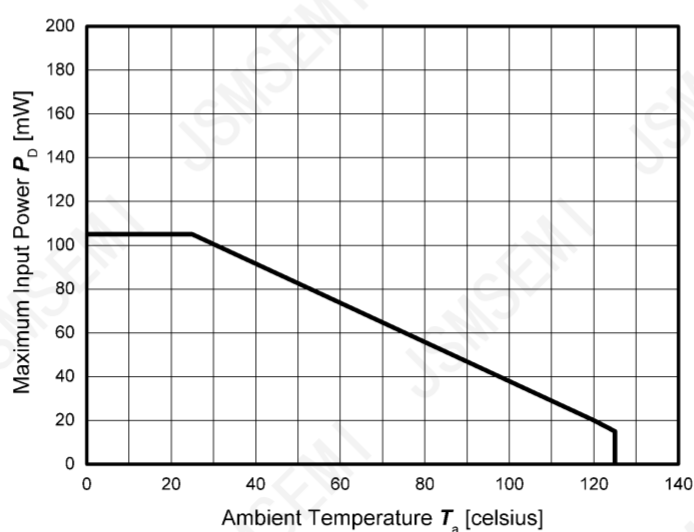
Figure 1. 最大输入功率-环境温度
