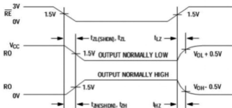
图 1 1 接收开启和关闭时间
