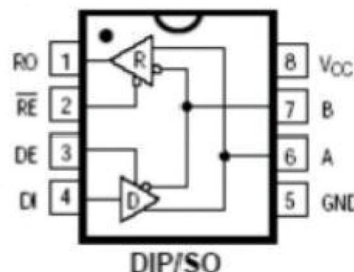
图1封装图
