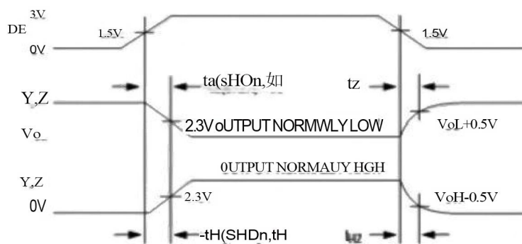
图10驱动开启和关闭时间
