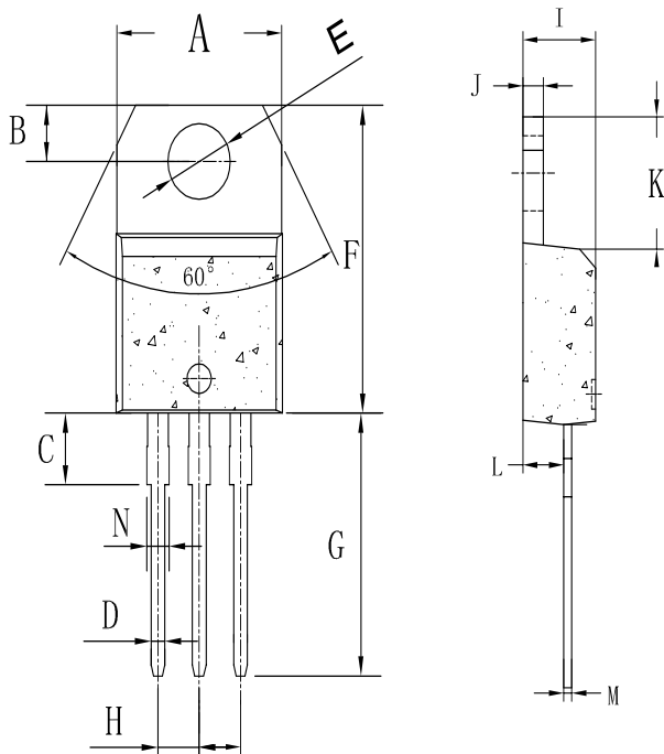
TO-220A
