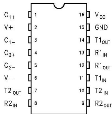
SOP-16/TSSOP-16
