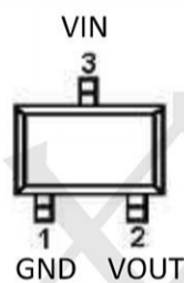
SOT23
