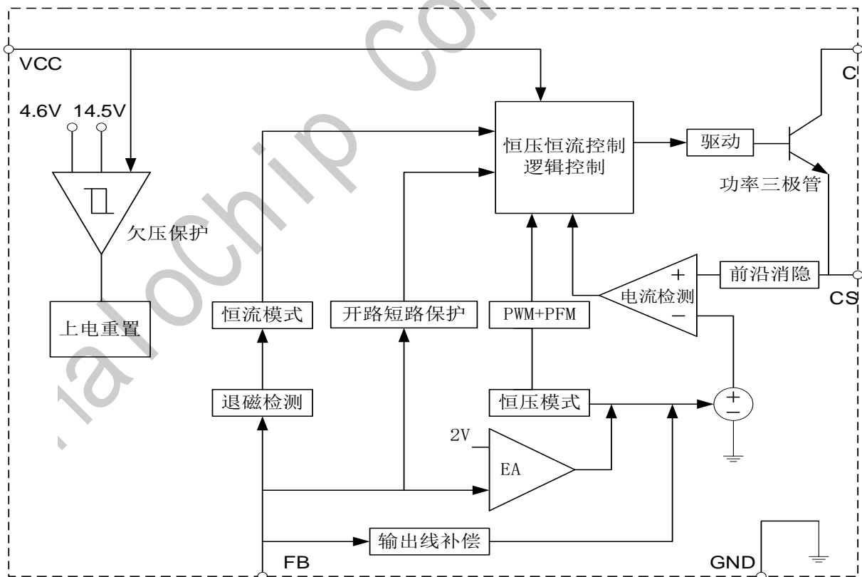
图 3 GP8675X 内部框图
