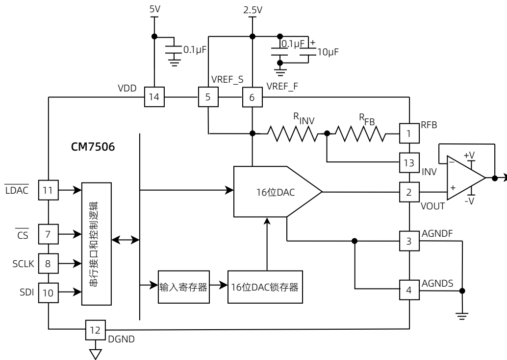
图 20 典型连接
