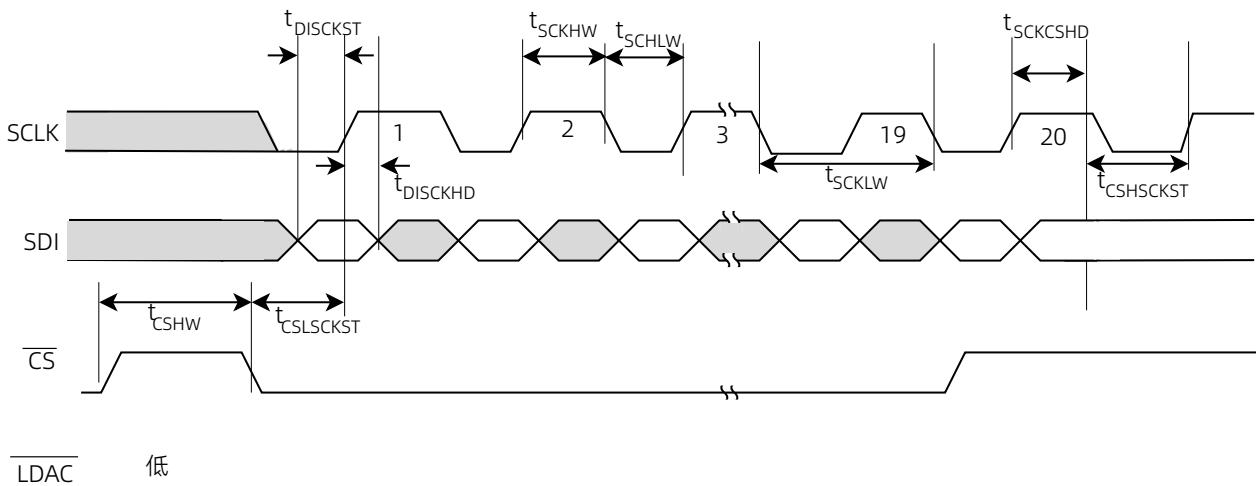
图 1 SPI 时序图
