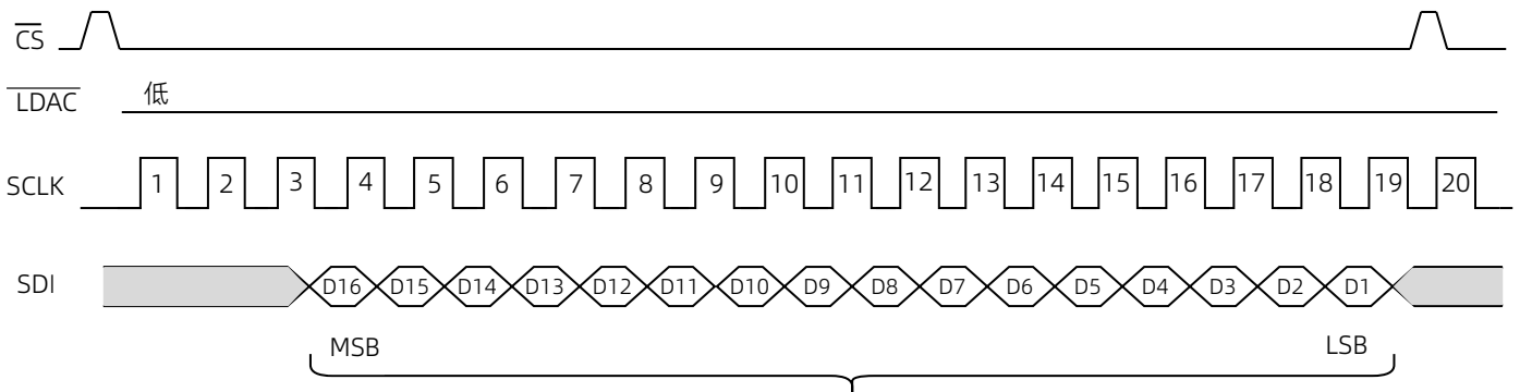
图 19 时序图
