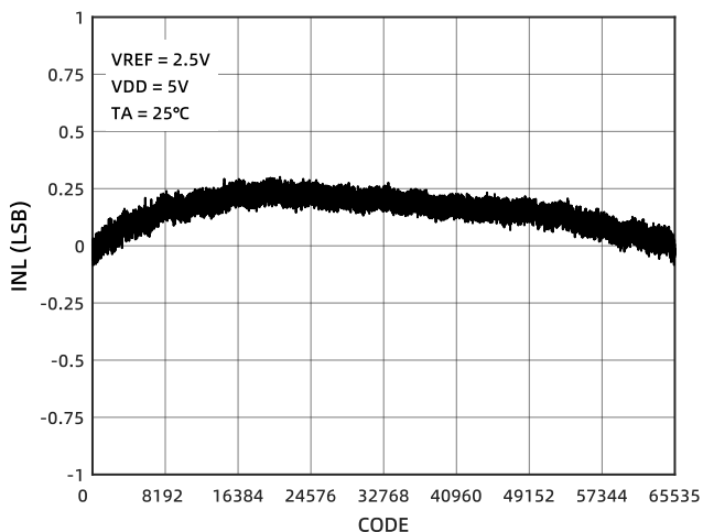
图 2 INL
