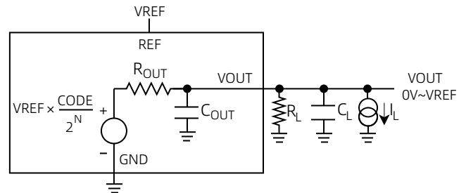
图 18 VOUT 管脚等效电路
