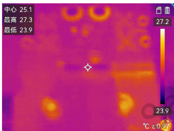
0A 温升表现
