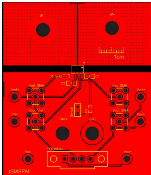
Demo 板正面
