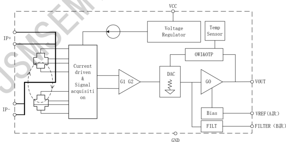
功能框图
