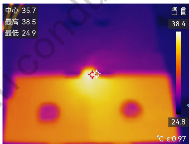
20A 温升表现
