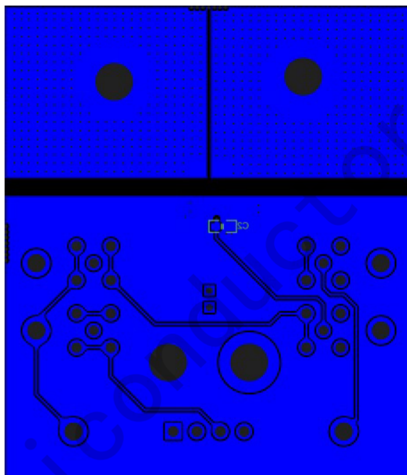
Demo 板反面
