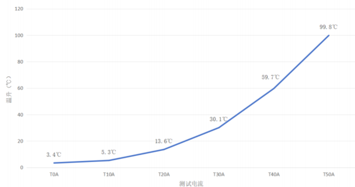
温升曲线图
