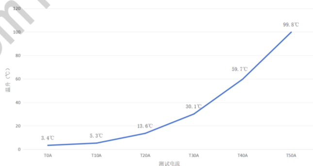
温升曲线
