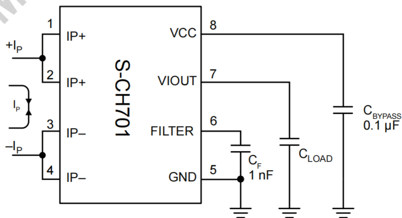
典型应用电路图
