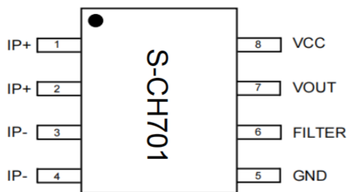
引脚图
