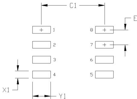
图 20.8 引脚SOP 封装焊盘图案
