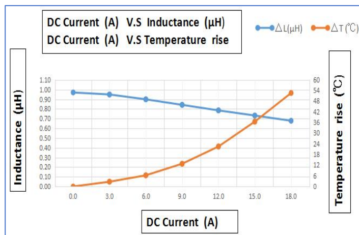
GSM0630-1R0-M
