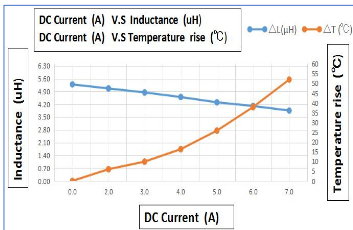
GSM0630-5R6-M
