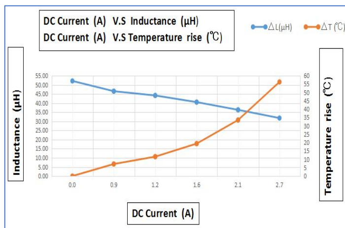
GSM0630-470-M
