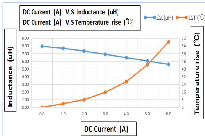
GSM0630-8R2-M
