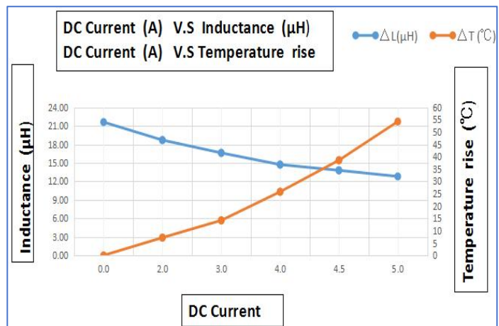
GSM0630-220-M
