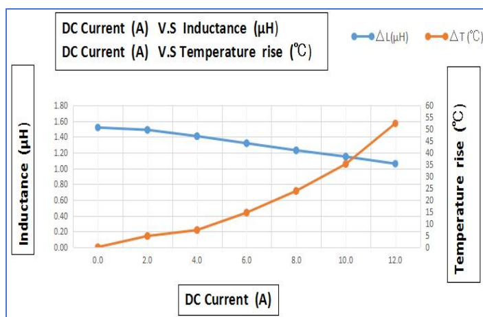
GSM0630-1R5-M
