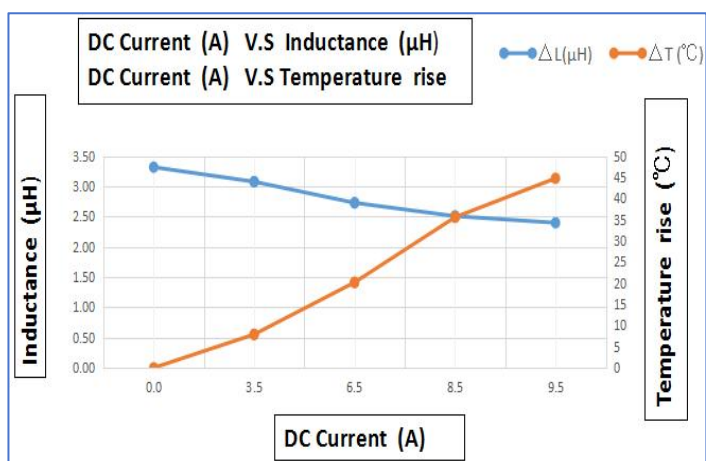
GSM0630-3R3-M
