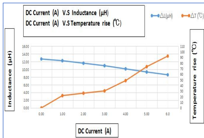
GSM0630-330-M
