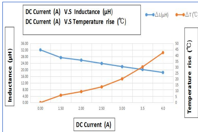
GSM0630-330-M
