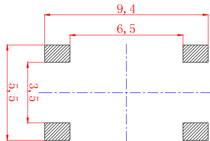
PCB参考图
