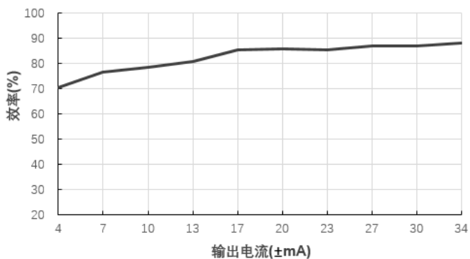
效率Vs输出电流( V_{in}=12V )@E1212S-1WR3
