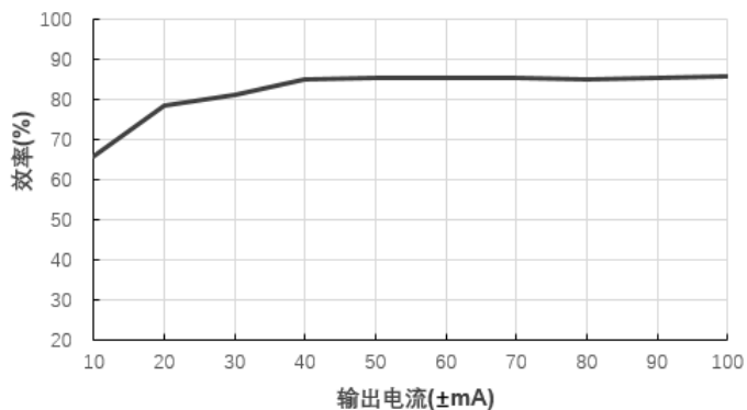
效率Vs输出电流( V_{in}=5V )@E0505S-1WR3
