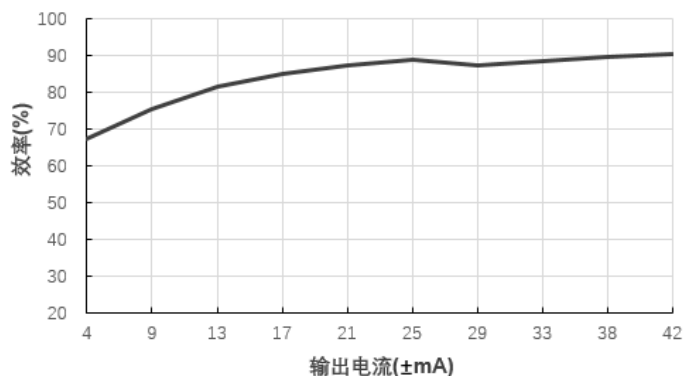
效率Vs输出电流(Vin=24V)@E2412S-1WR3
