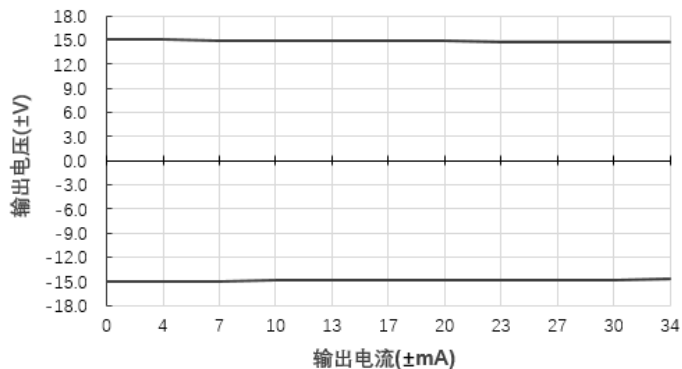
输出电压Vs输出电流( V_{in}=24V )@E2415S-1WR3
