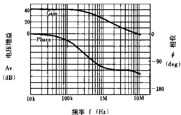
电压增益、相位与频率
