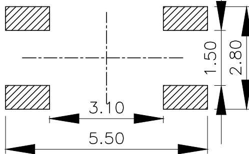
PCB. 焊接图
