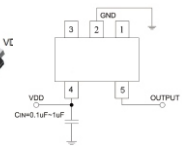
SOT-553
