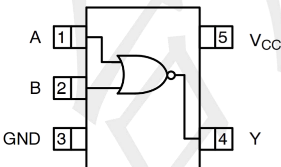
SOT353
