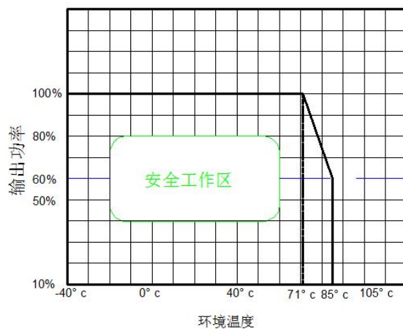
温度曲线图
