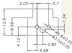
2P PCB 安装尺寸
