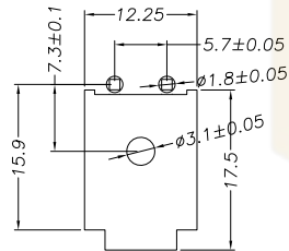
2P PCB 安装尺寸
