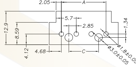
3-8P PCB 安装尺寸
