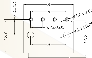
3-8P PCB 安装尺寸
