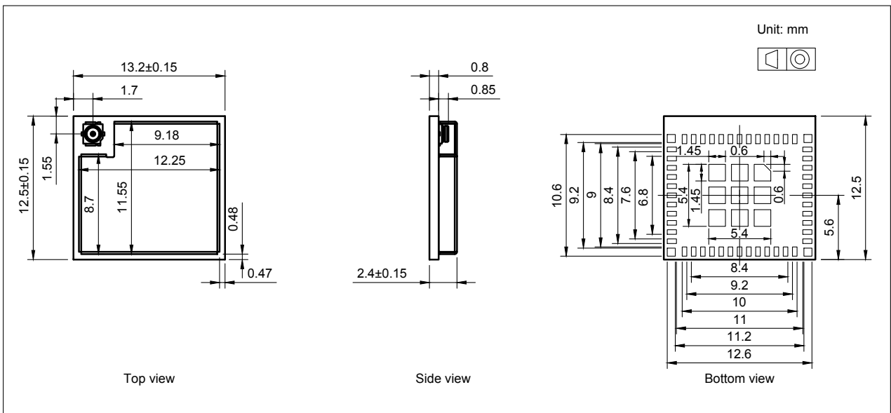
图 9: ESP8684-MINI-1U 尺寸
