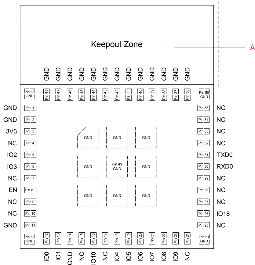
图 3: ESP8684-MINI-1 管脚布局 (顶视图)
