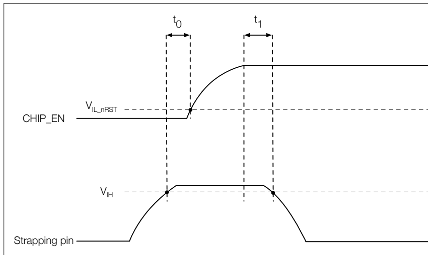
图 4: Strapping 管脚的时序参数图
