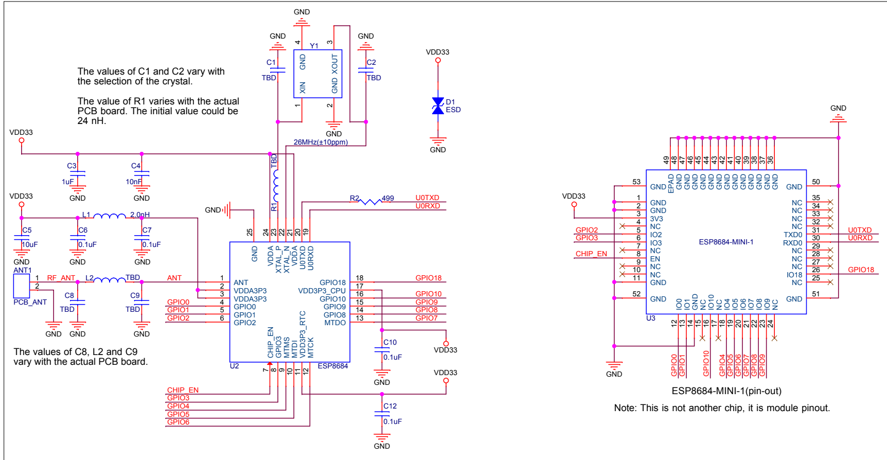
图 5: ESP8684-MINI-1 原理图
