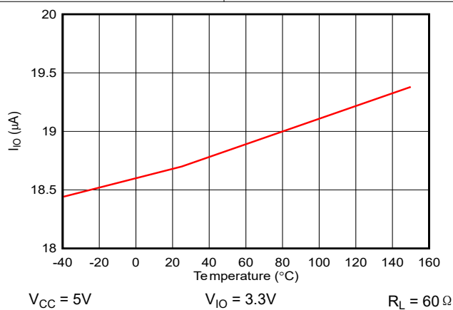
图 5-3. I_{IO} 待机电流与温度间的关系
