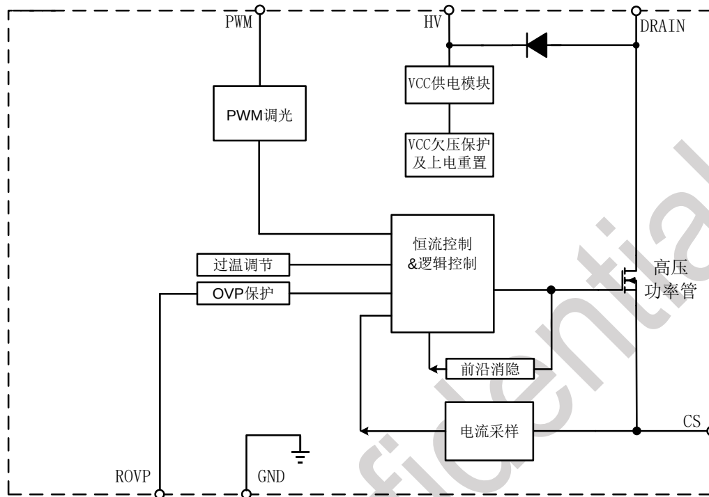
图 3 BP2881X 内部框图
