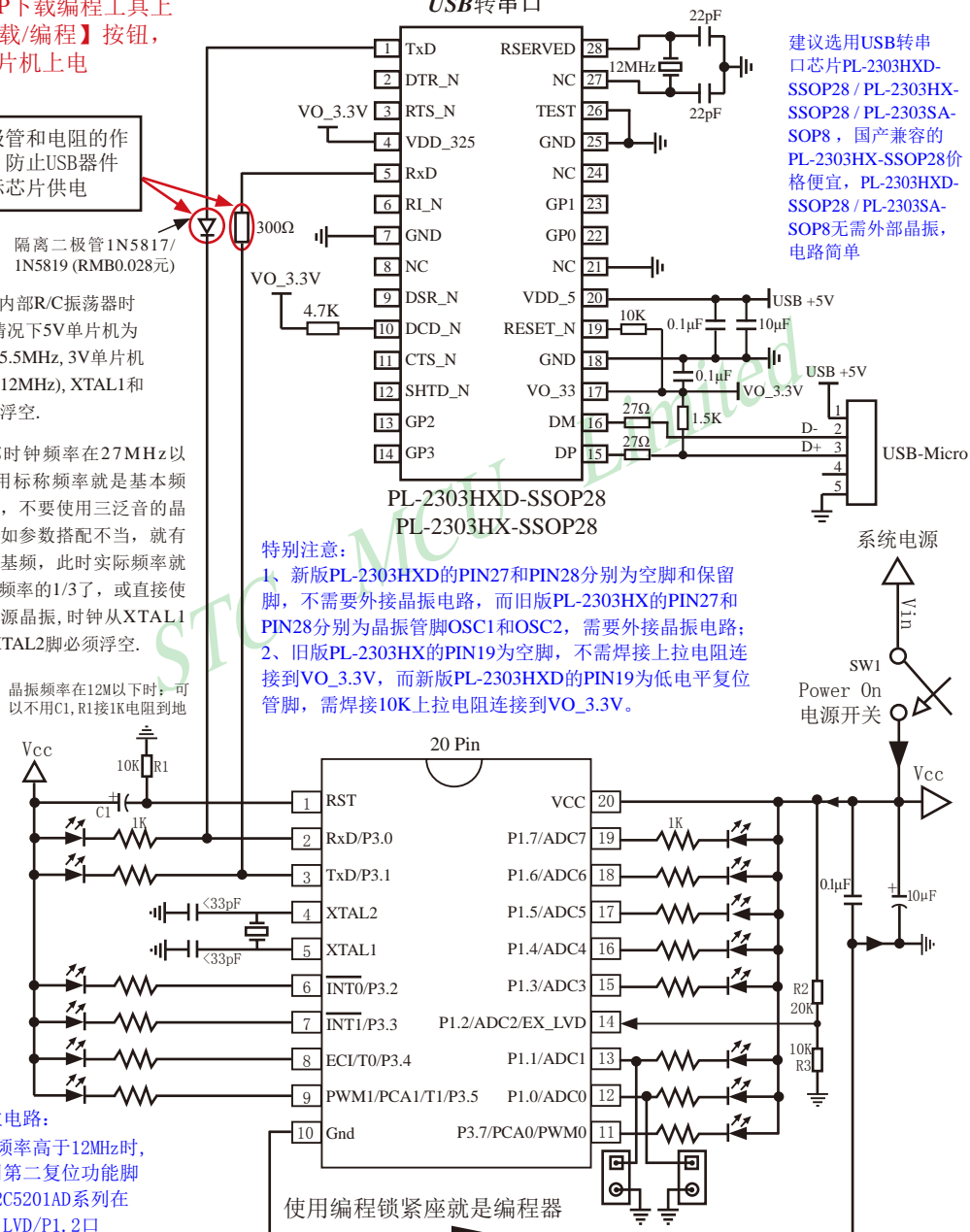
STC 单片机在线编程线路 USB转串口
