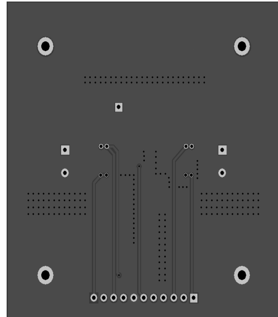
Bottom Layer
