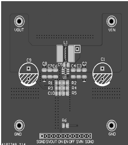
Top Layer
