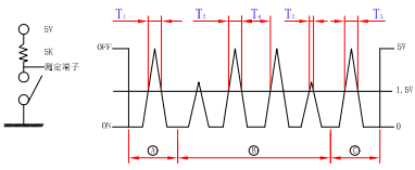
操作示意图
