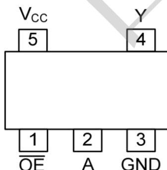
SOT353
