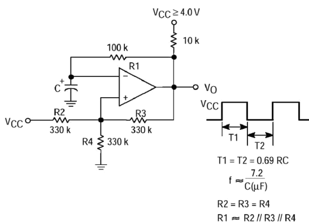
方波振荡器
