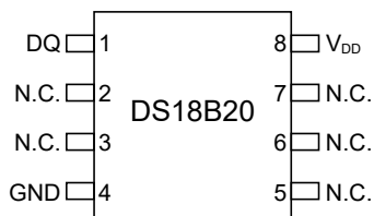
MSOP8
