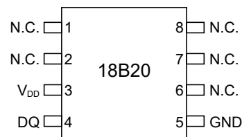
SOP8
