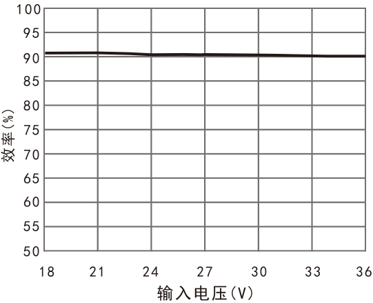
效率Vs输入电压(满载) VRB2405LD-15WR3
