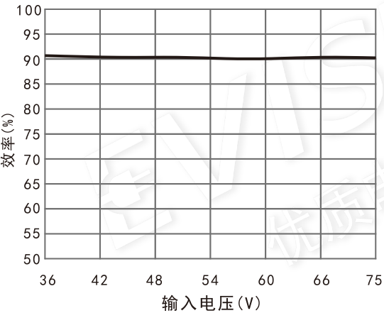
效率Vs输入电压(满载) VRB4815LD-15WR3
