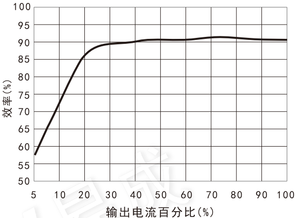
效率Vs输出负载(Vin=24V) VRB2405LD-15WR3
