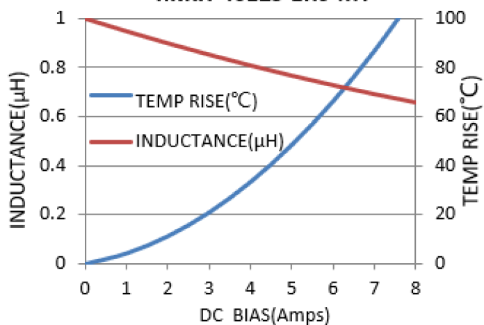
HNRA-4012S-1R0-MT
