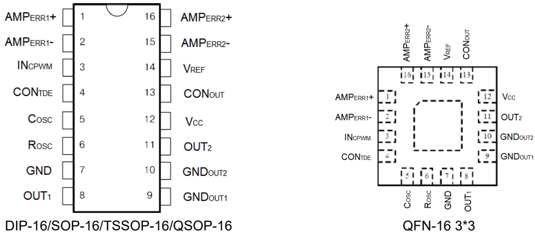
图 2 KA7500B 管脚 (顶部视图)
