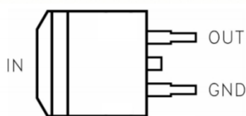
TO-263-2
