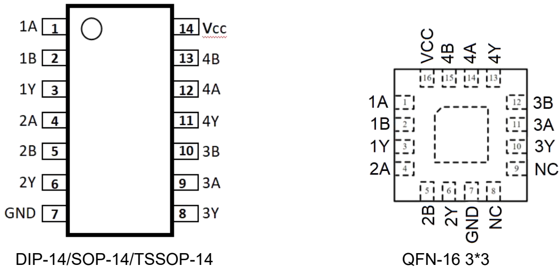
图 3、74HC00 引脚排列图
