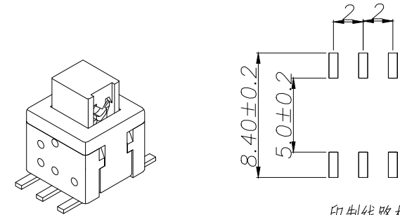
印制线路板 PCB Layout Recommended
