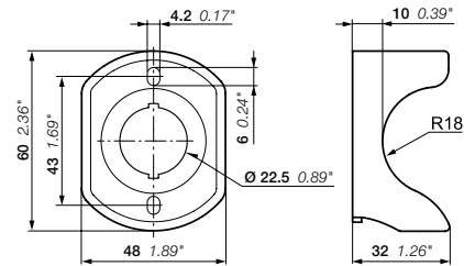
CA1 尺寸 (mm, 英寸)
