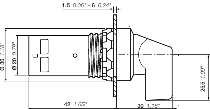
C3SS, 长手柄操作
