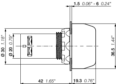
CP6 尺寸 (mm, 英寸)
