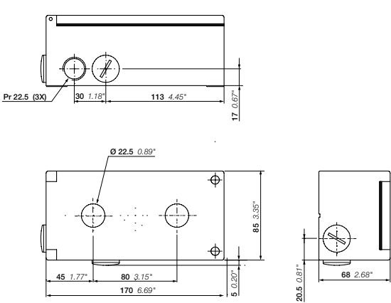
2底座和3底座KEM2-0、KEM3-0
