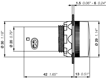
CB1 尺寸 (mm, 英寸)
