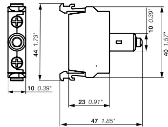
MLBL 尺寸 (mm, 英寸)
