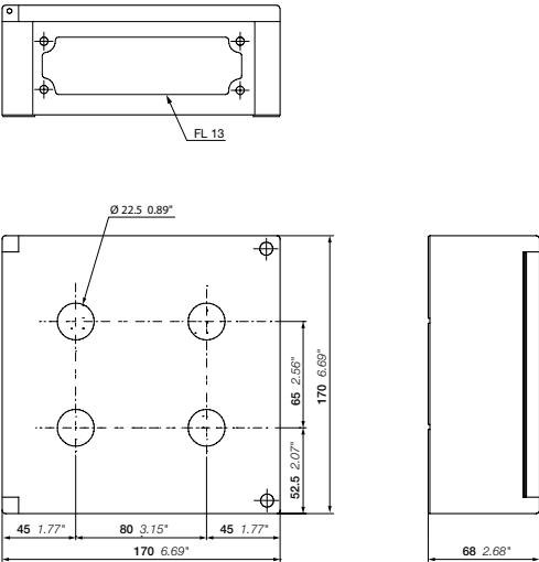
4或6底座KEM4-0、KEM6-0
