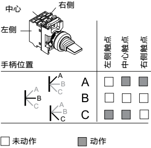
触点状态, 3位置
