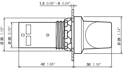
C2SS, 短手柄操作 尺寸 (mm, 英寸)
