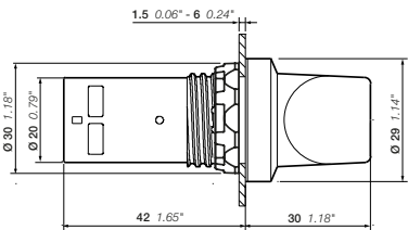
C3SS, 短手柄操作
