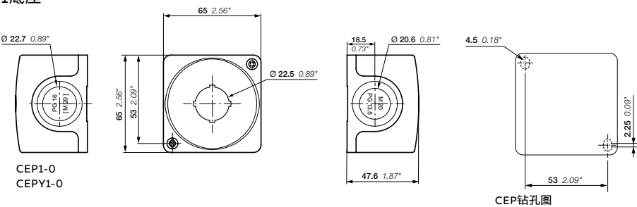
CEP钻孔图
