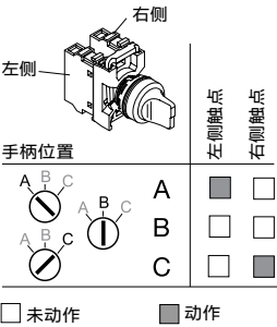
触点状态
