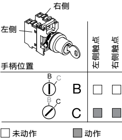
触点状态
