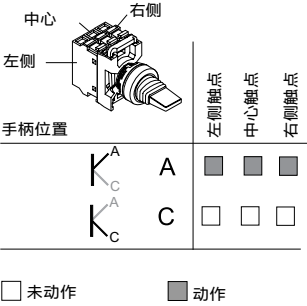
触点状态, 2位置
