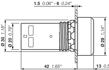
CP1 尺寸 (mm, 英寸)
