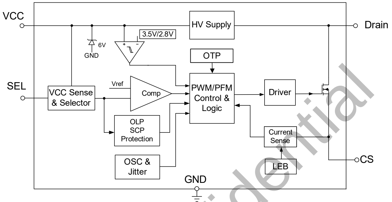
图 4 BP2525BC 内部框图
