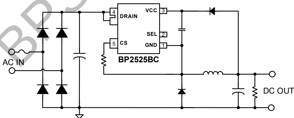
图 1 BP2525BC 典型应用
