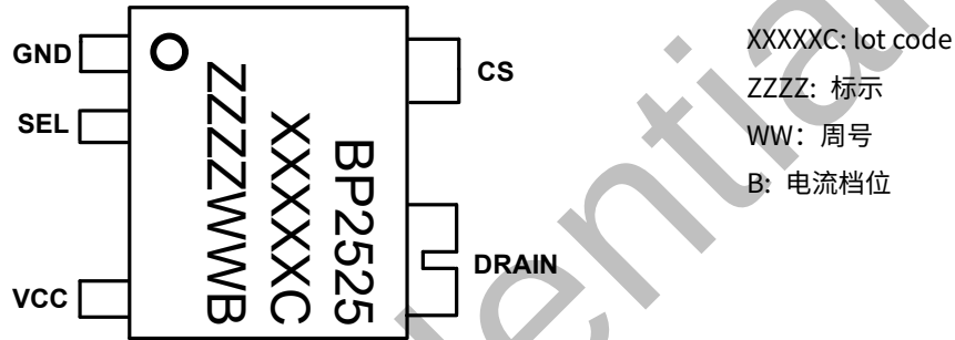
图 2 管脚封装图
