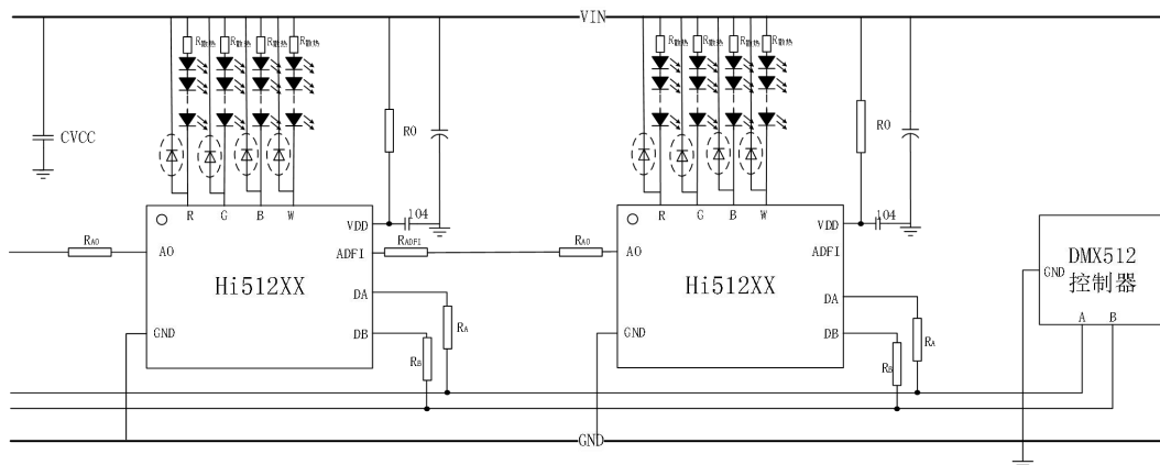
图 11.1.1 典型应用方案 1
