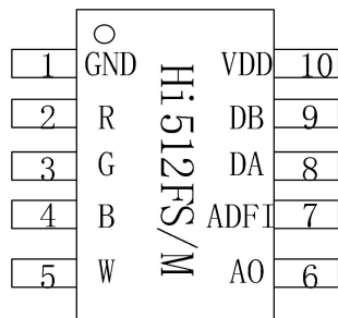
图 5.1 管脚图
