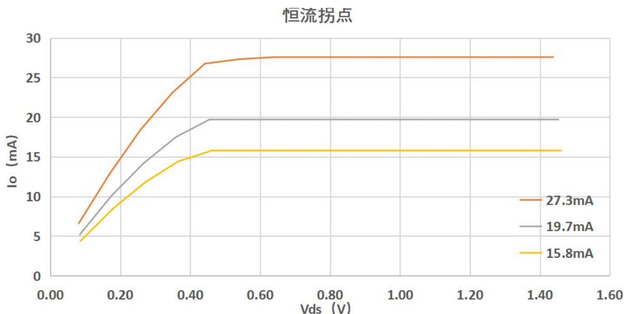
图 10.1 恒流拐点
