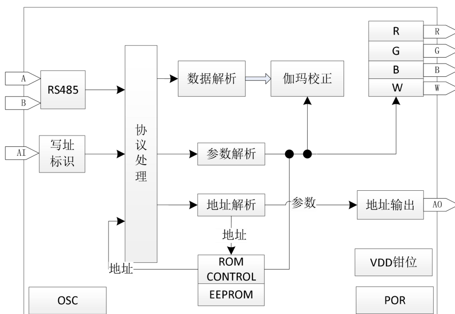
图 6.1 结构原理框图
