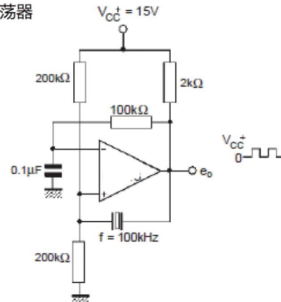
方波振荡器
