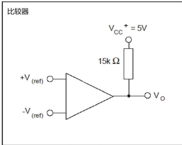
驱动TTL
