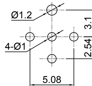
P. C. B. LAYOUT
