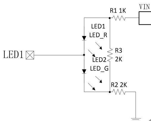
图 5 LED指示灯原理图。
