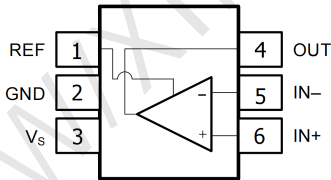
SC70-6(SOT-363)
