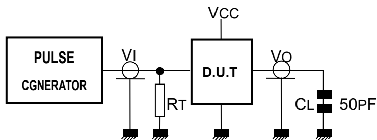
图 5、交流测试图
