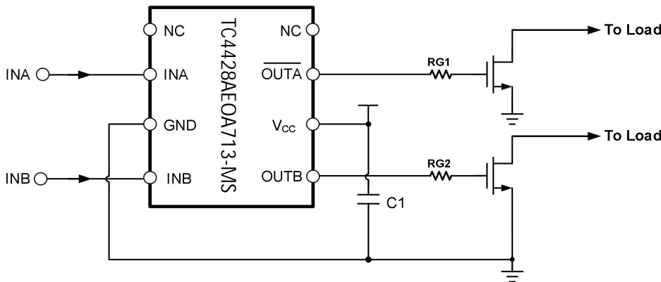
TC4428AEOA713-MS 典型应用电路图
