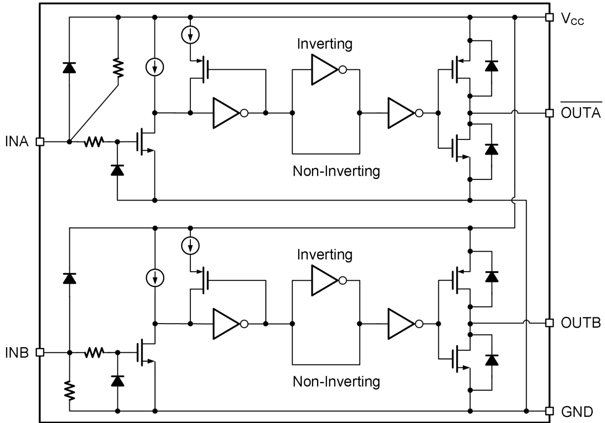
TC4428AEOA713-MS 功能框图
