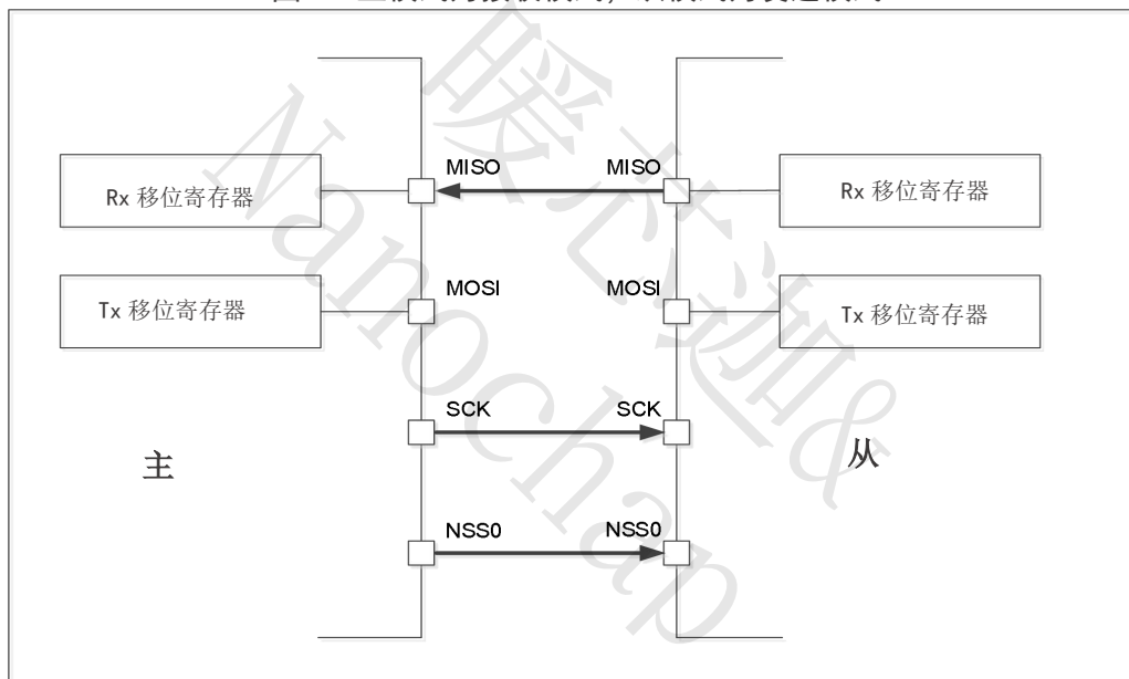
图 12 主模式为接收模式，从模式为发送模式
