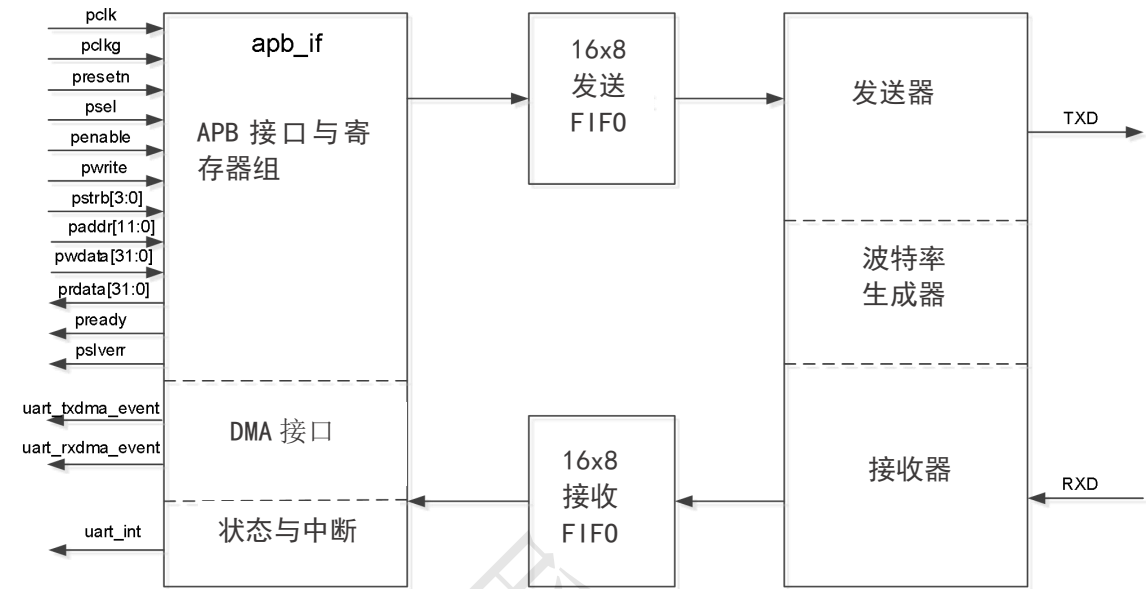
图 16 UART 框图
