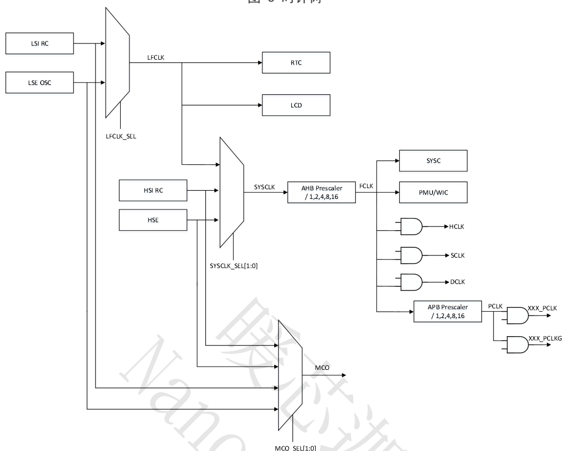
图 6 时钟树
