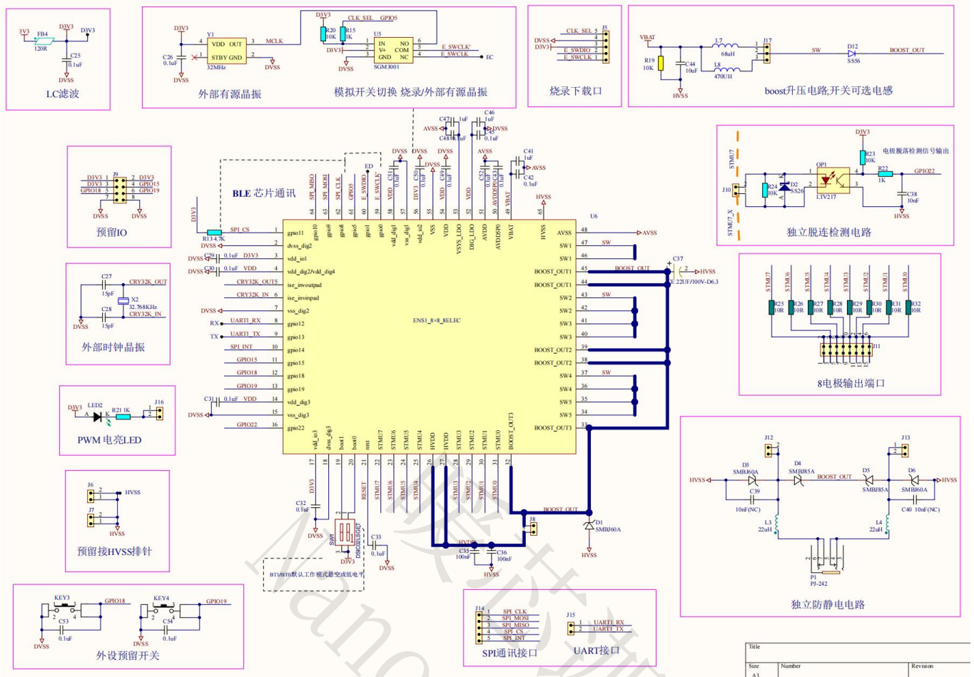
图 32 原理图 3/3
