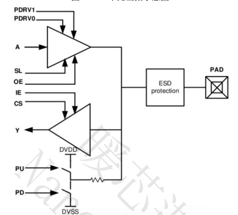
图 7 I/O 单元函数示意图
