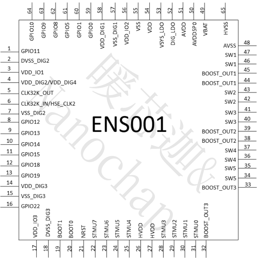
图 2 芯片原理图
