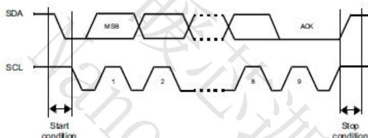
图 18 I2C 总线协议
