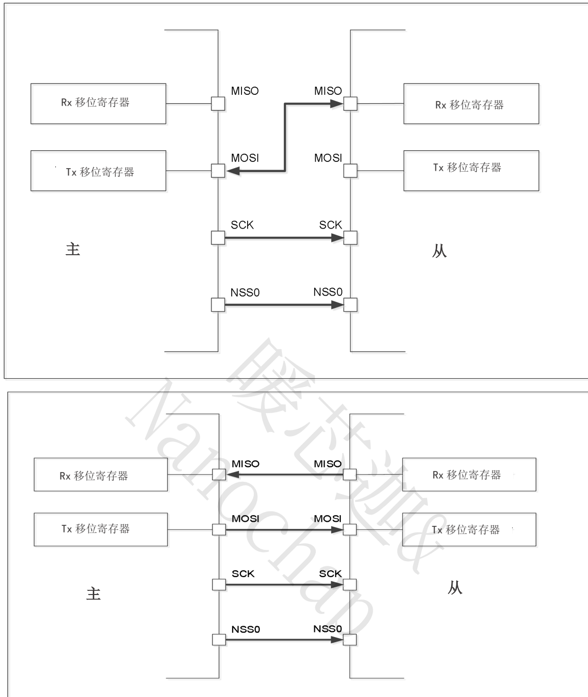
图 10 半双工传输应用
