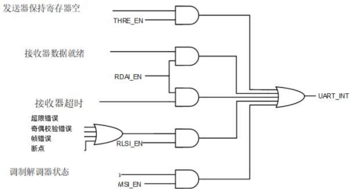
图 17 UART 中断输出
