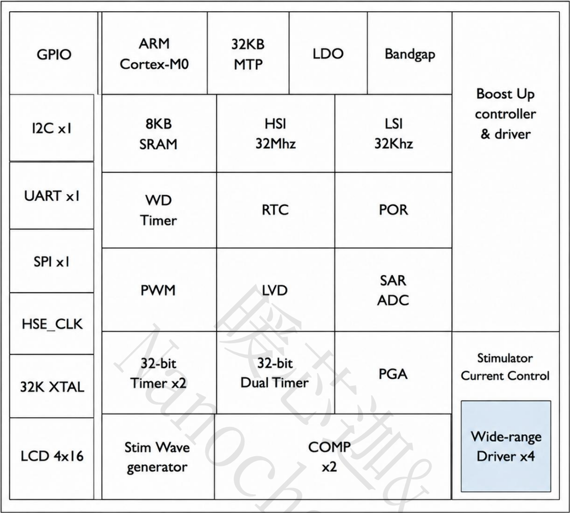
图 1 原理框图
