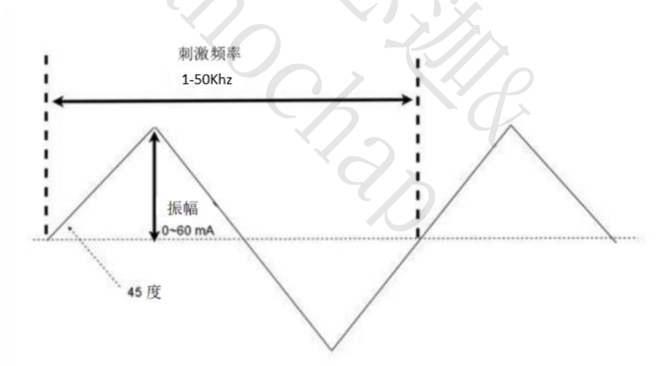
图 29 三角波形
