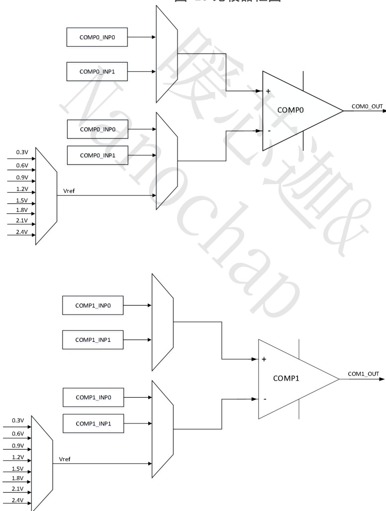
图 25 比较器框图
