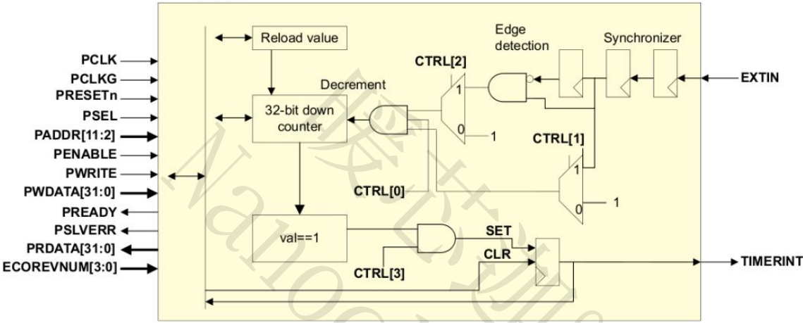
图 23 定时器框图
