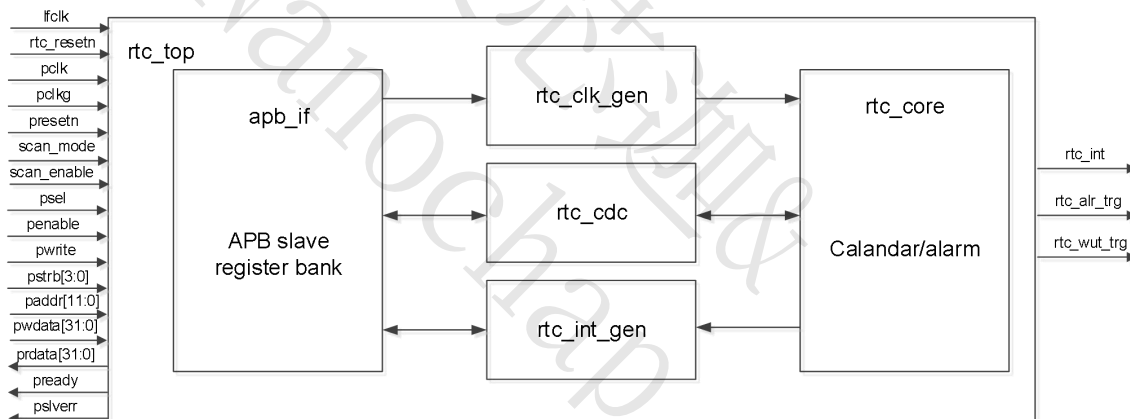
图 20 RTC 框图
