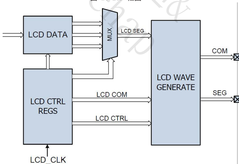
图 26 LCD 框图
