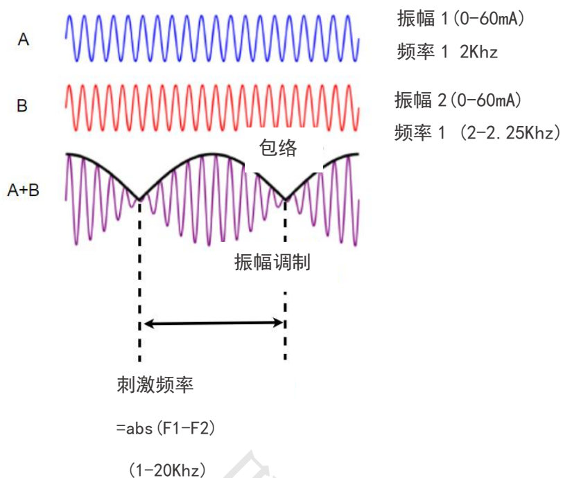
图 28 正弦波形
