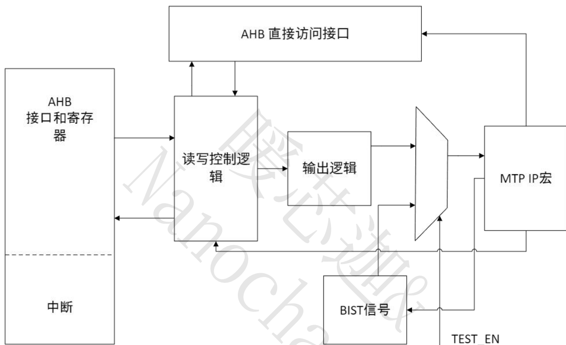
图 5 MTP 框图
