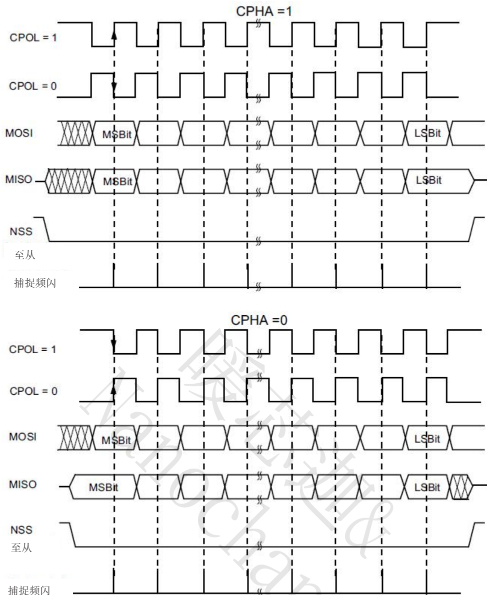
图 15 数据时钟时序图
