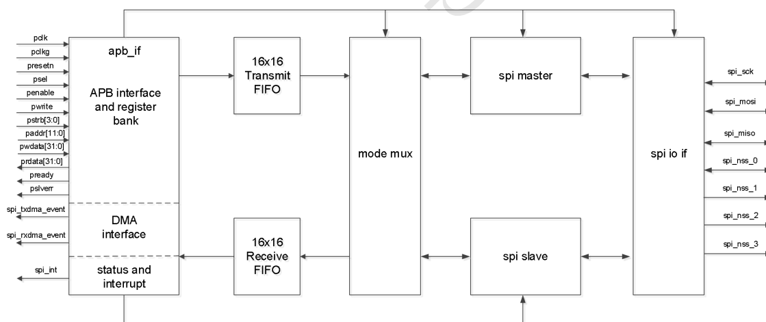
图 8 SPI 框图
