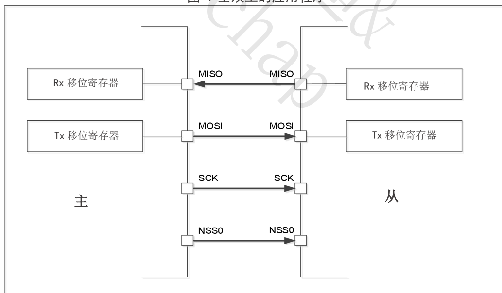
图 9 全双工的应用程序
