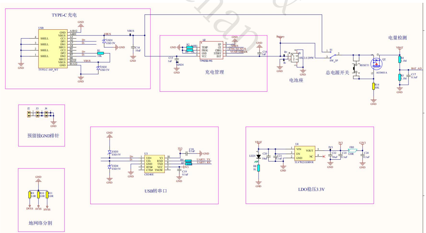
图 32 原理图 3/3
