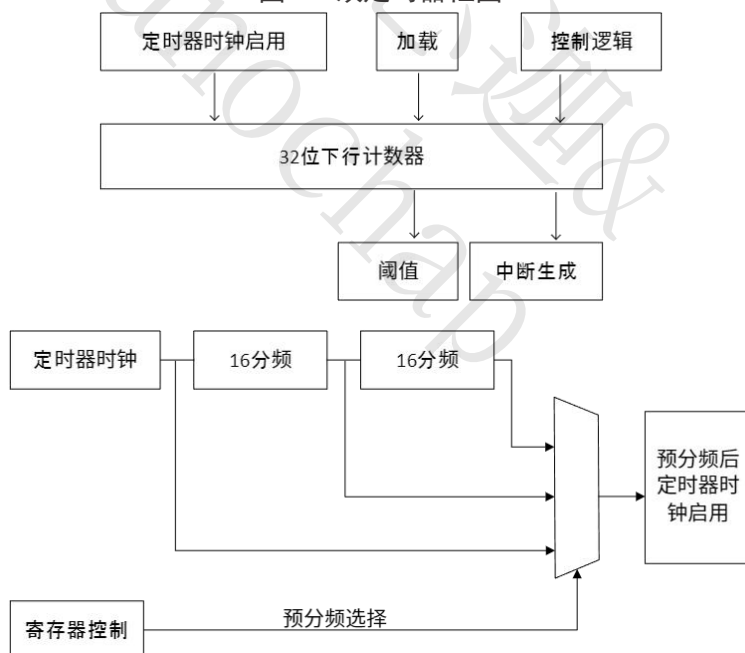
图 24 双定时器框图
