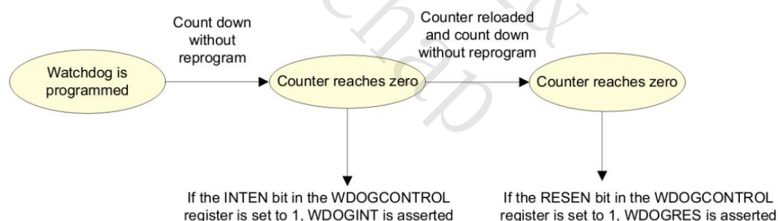
图 21 WDT 流程图
