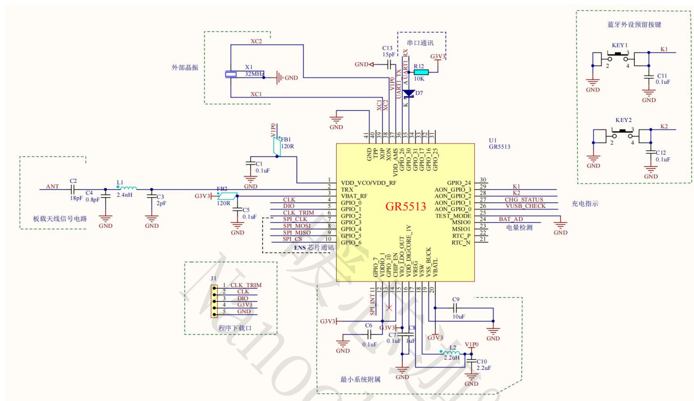
图 30 原理图 1/3
