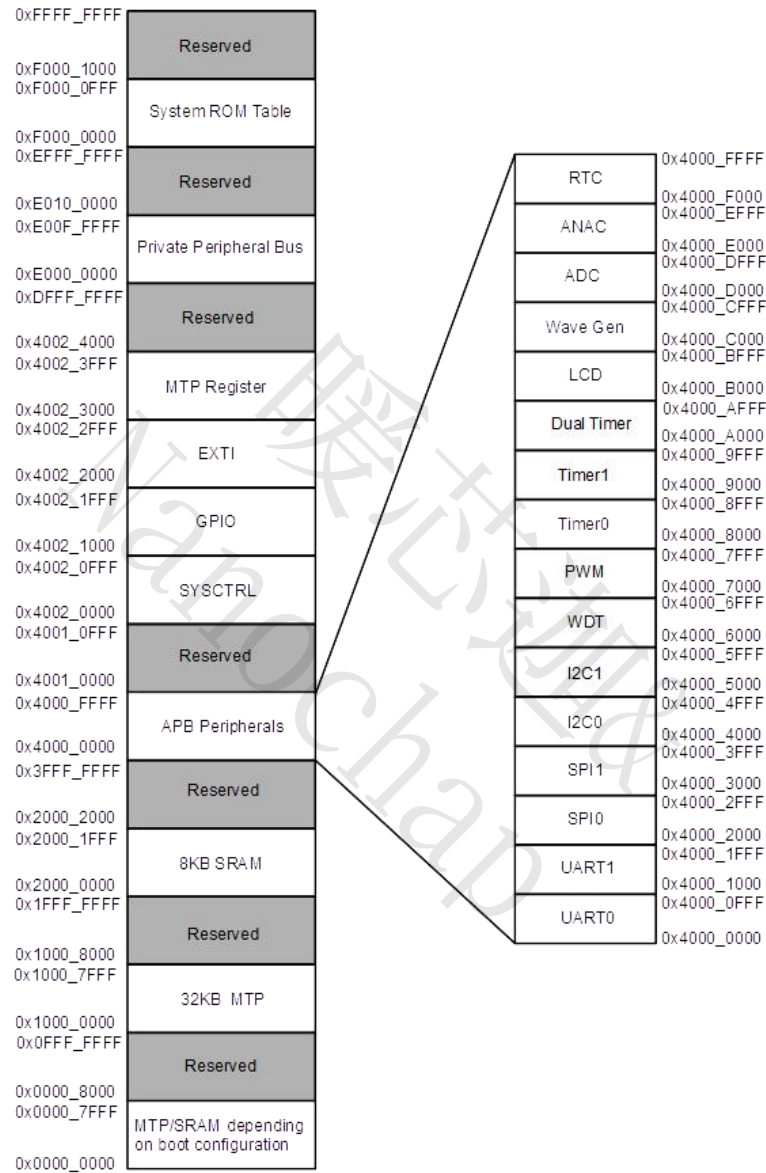
图 4 内存映射图
