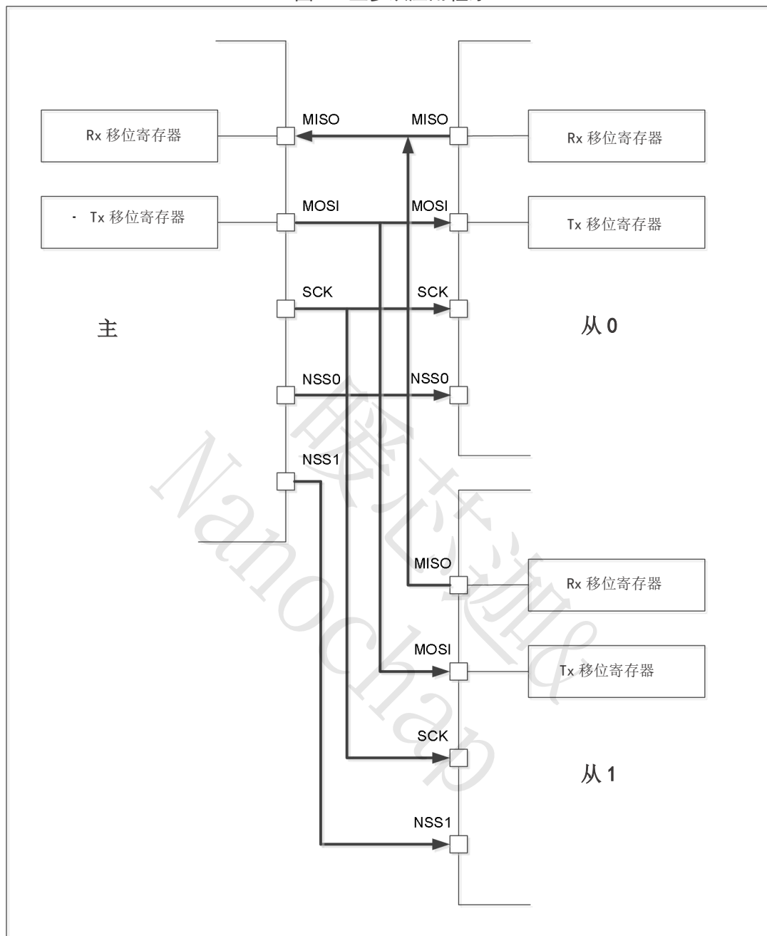
图 13 主多从应用程序
