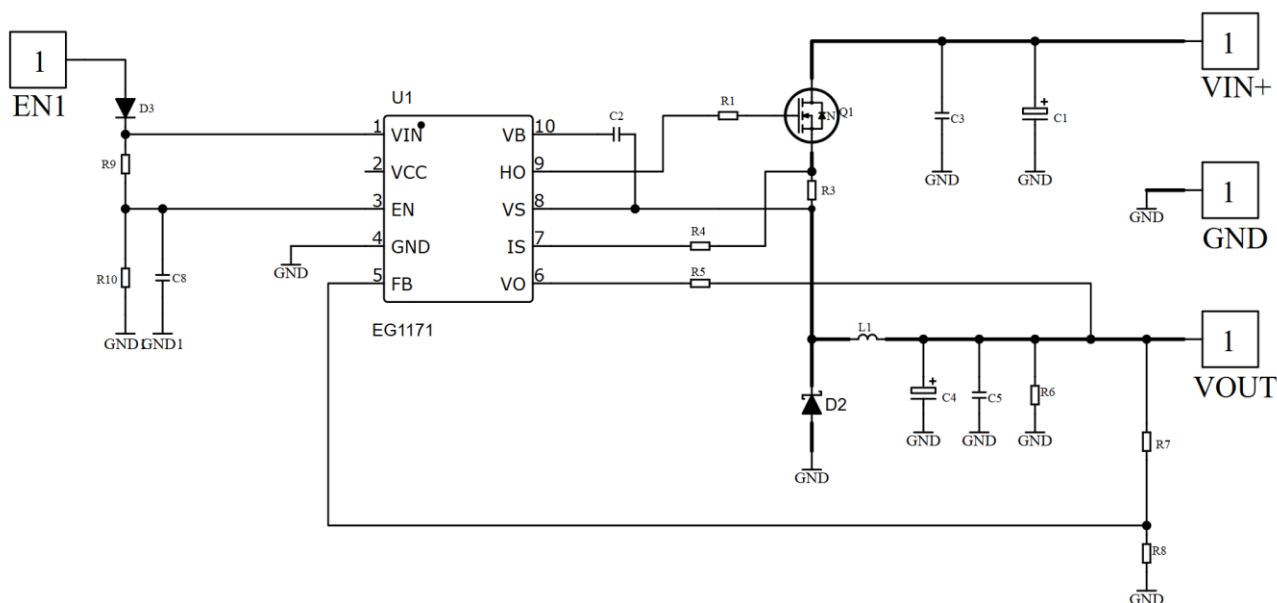
图 6-5. EG1171 12V 输出关闭延时典型应用图
