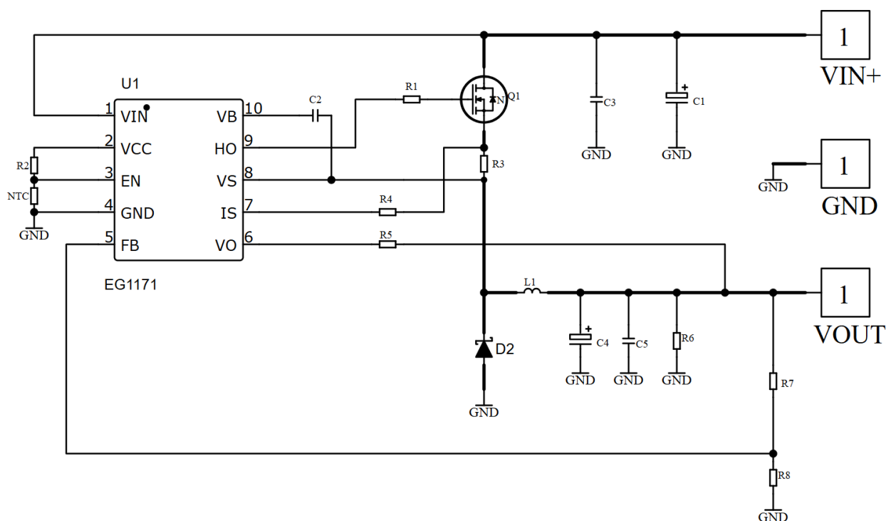
图 6-3. EG1171 12V 输出外置温度保护典型应用图
