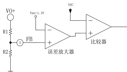
图 8.1 EG1171 输出电压调整电路
