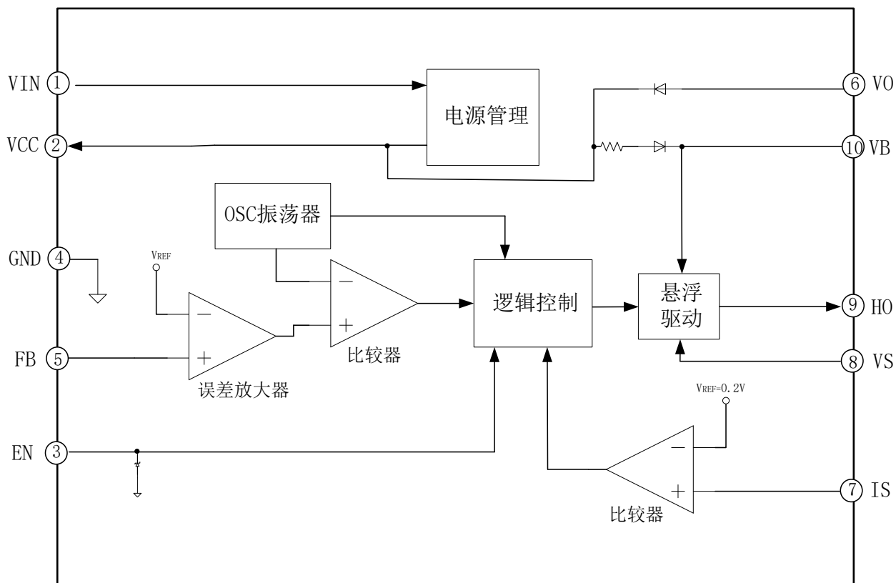
图 5-1. EG1171 内部电路图
