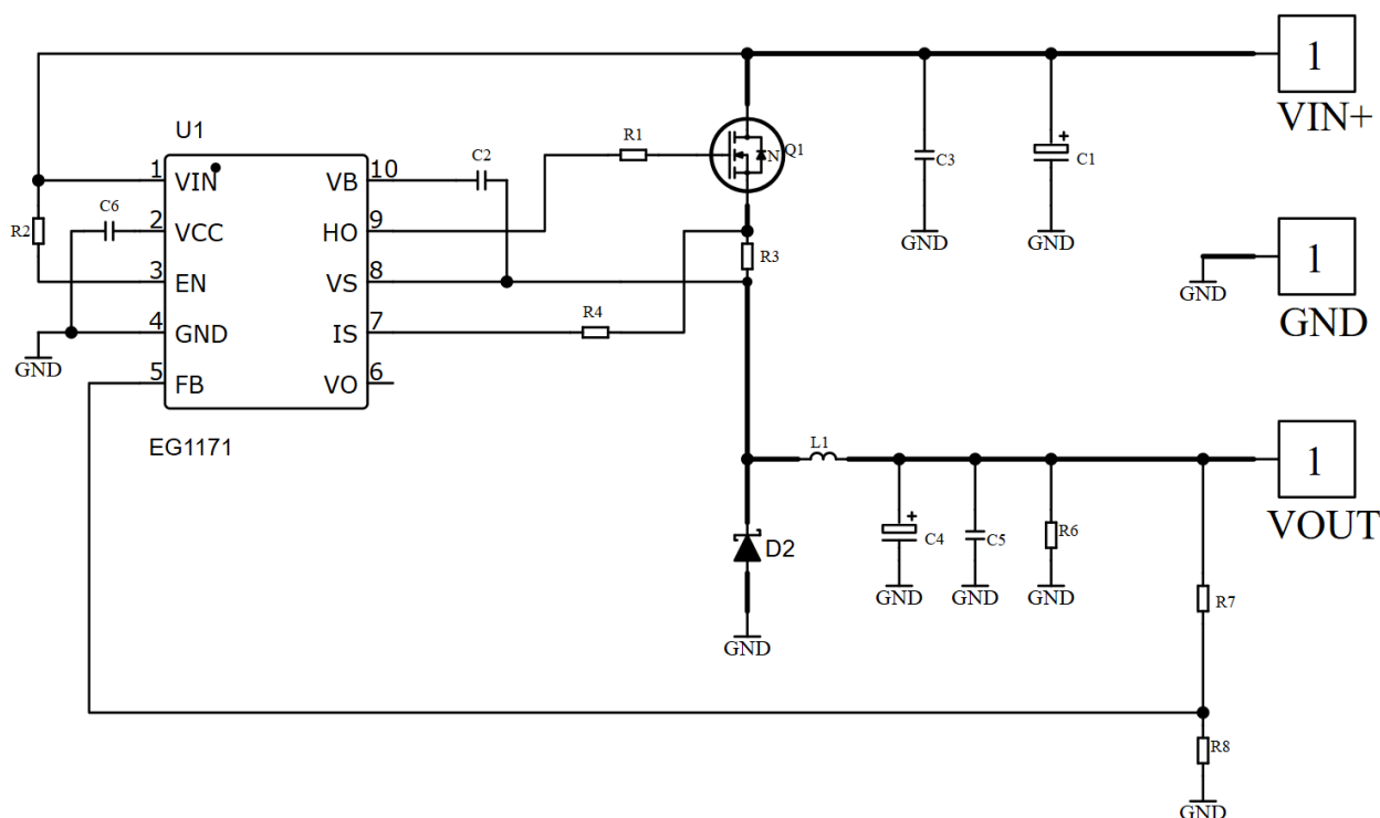
图 6-1. EG1171 5V 输出及小功率场合典型应用图
