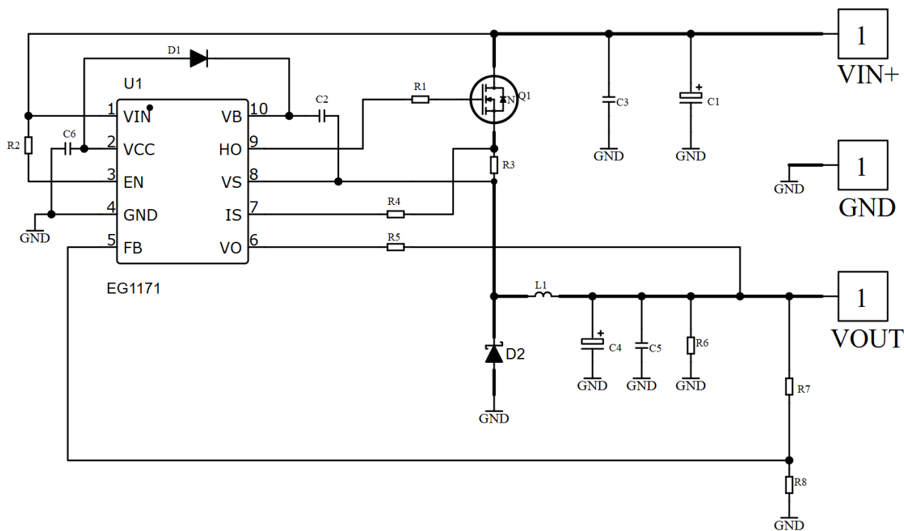
图 6-4. 输出 12-15V 场合，外置自举二极管输出反馈典型应用图
