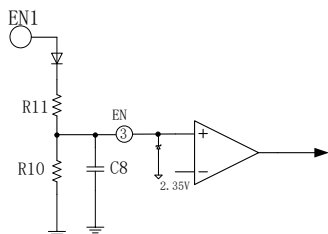
图 8.2 EG1171 关闭延时电路
