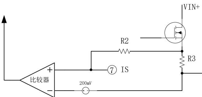
图 8.3 EG1171 峰值限流电路
