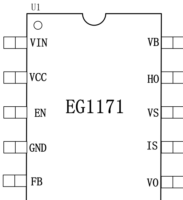
图 4-1. EG1171 管脚定义
