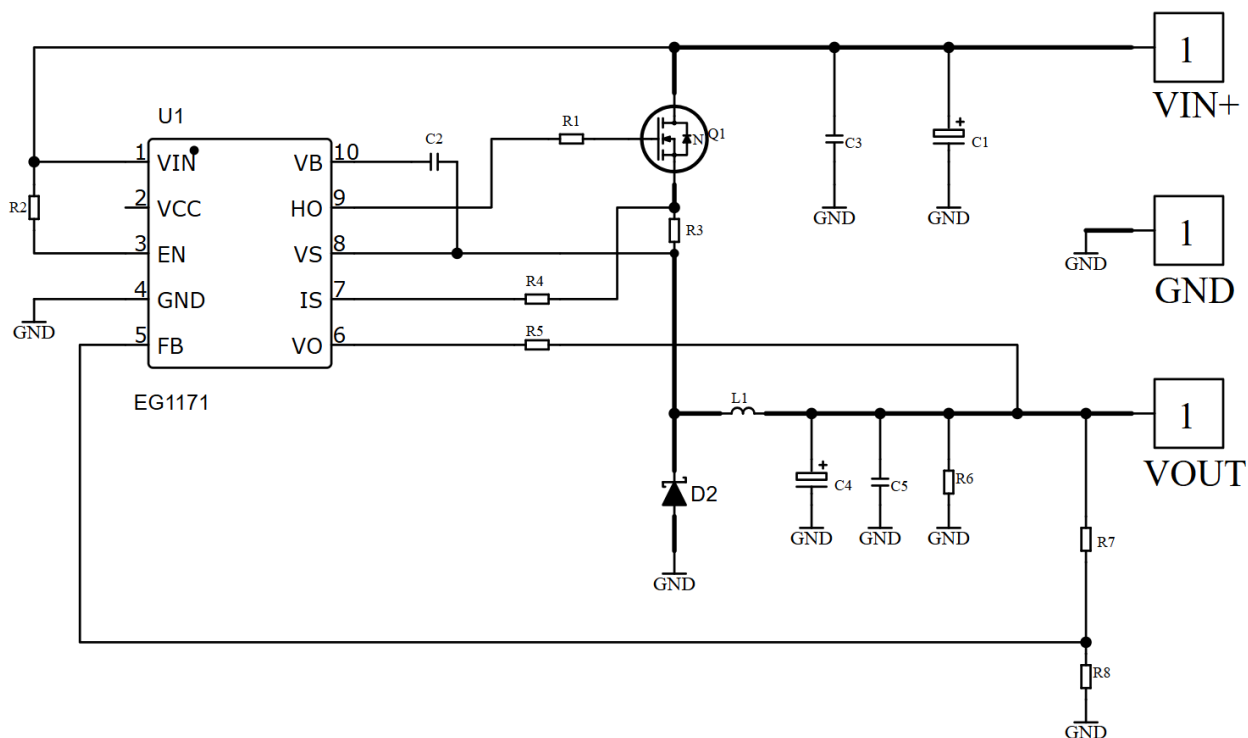
图 6-2. EG1171 12V 输出小功率场合输出反馈典型应用图
