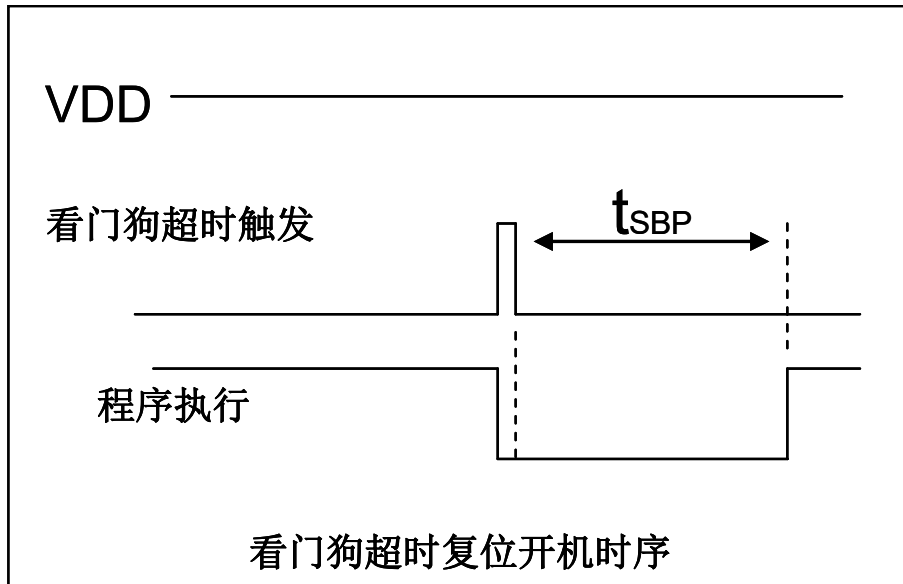
图 19: 看门狗超时溢出时序图
