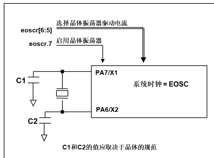
图 2: 晶体振荡器的的硬件连接
