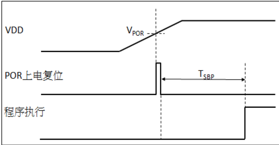
图 1：上电复位时序
