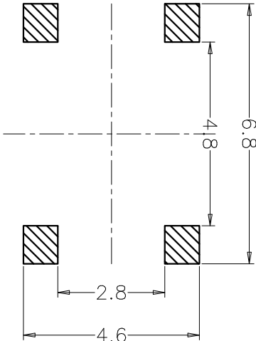
PCB. 焊接图
