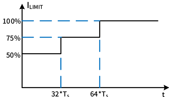
图 6. 软启动过程
