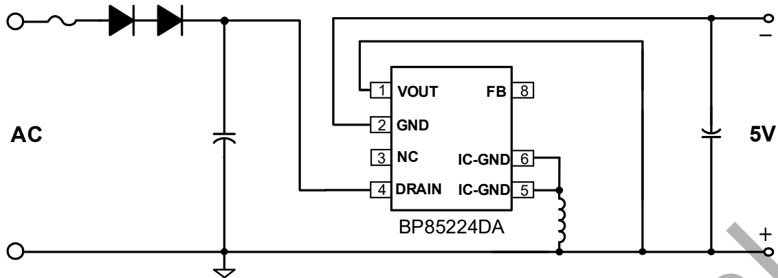
图 2. BP85224DA 典型 Buck-Boost 应用电路
